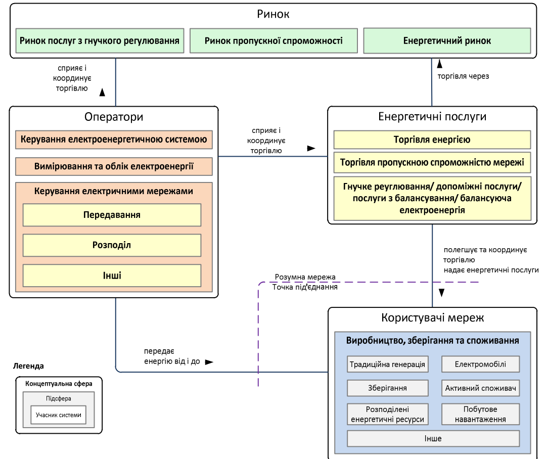
Європейська концептуальна модель Smart Grid
