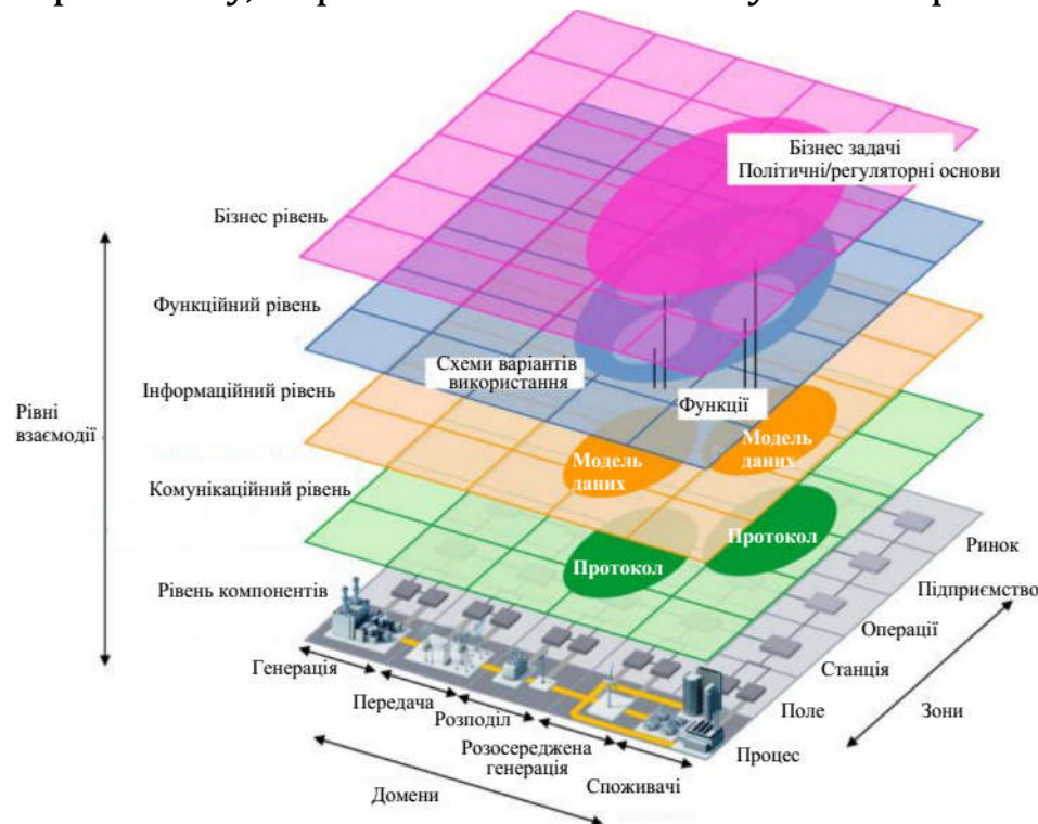
Базова модель архітектури Smart Grid
